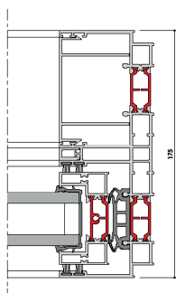
Coupe latéral
