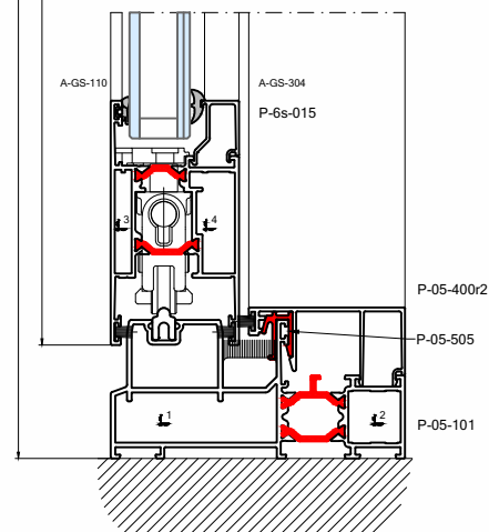
4_vleugelig_hefschuifraam_monorail
