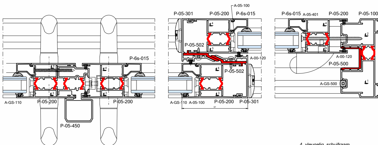
4_vleugelig_schuifraam
