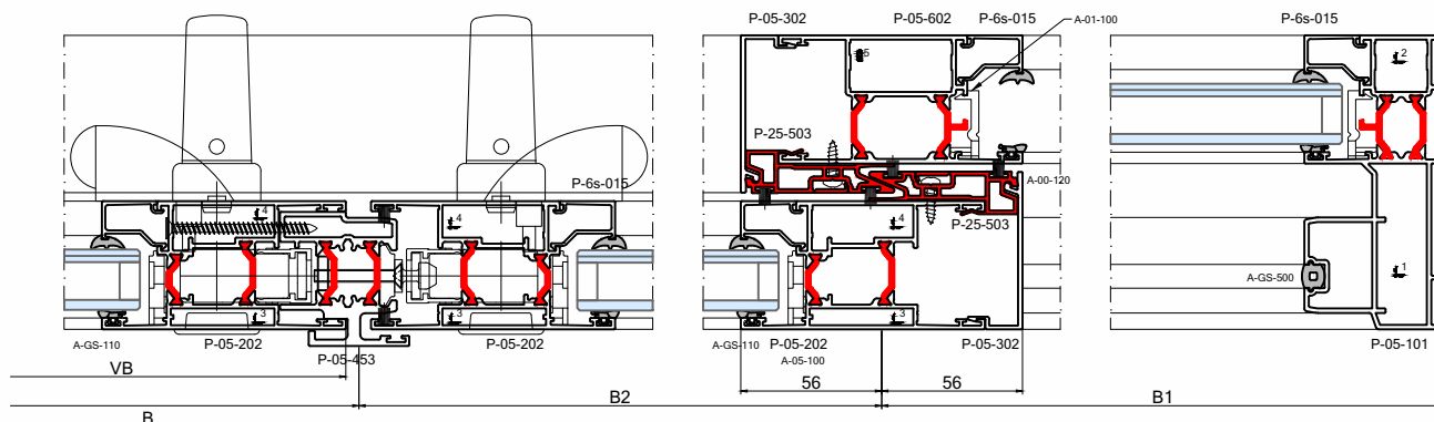
4_vleugelig_hefschuifraam_monorail
