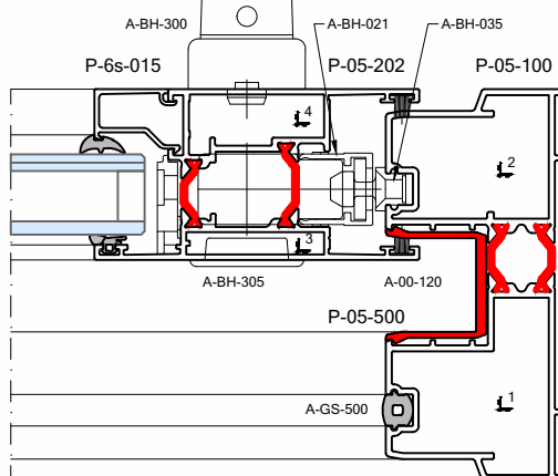
2_vleugelig_hefschuifraam
