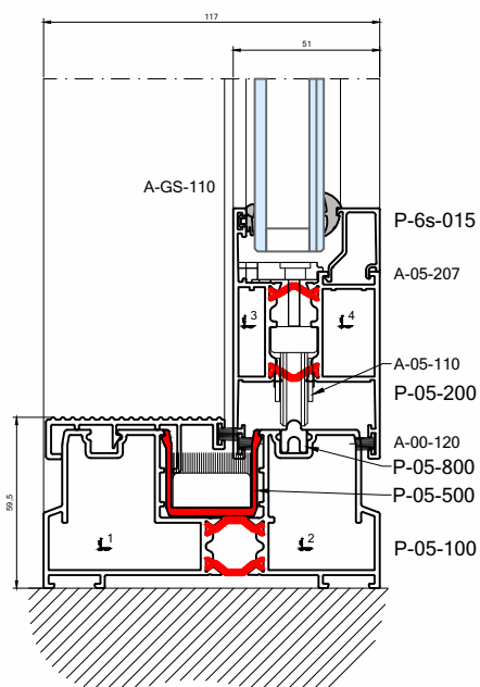
3_vleugelig_schuifraam_350
