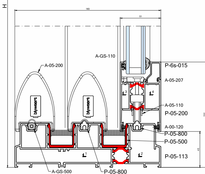
3_vleugelig_schuifraam
