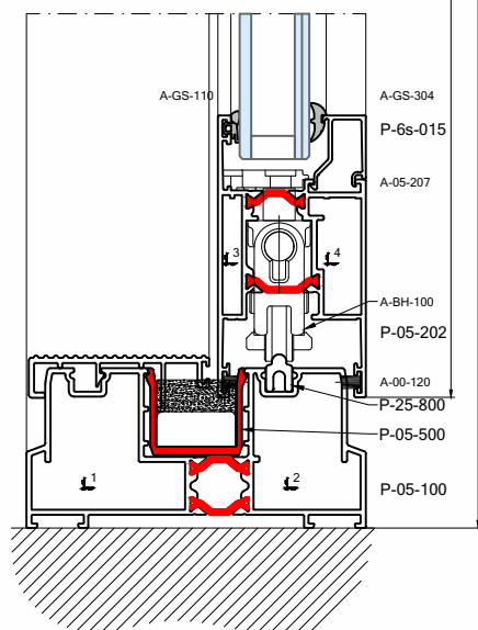
3_vleugelig_hefschuifraam_350
