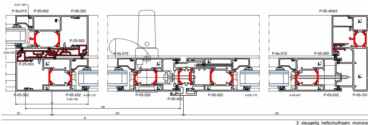
3_vleugelig_hefschuifraam_monorail
