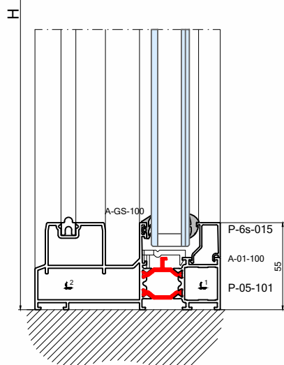
3_vleugelig_schuifraam_monorail
