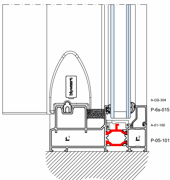
2_vleugelig_hefschuifraam_monorail
