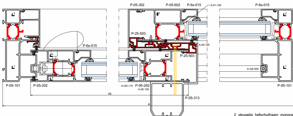
2_vleugelig_hefschuifraam_monorail
