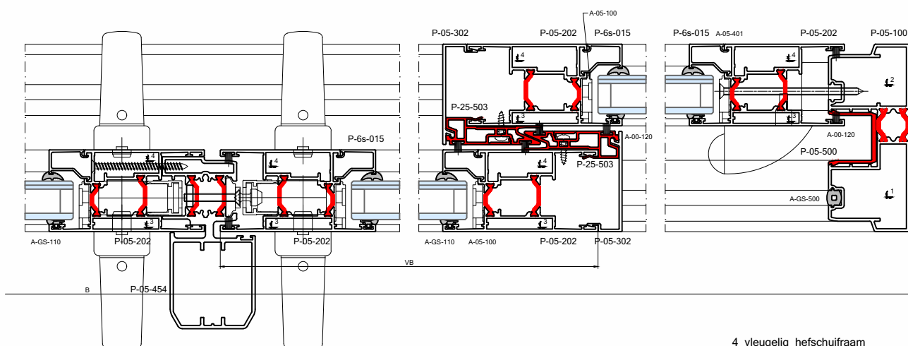
4_vleugelig_hefschuifraam
