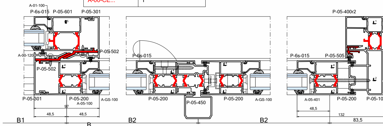
3_vleugelig_schuifraam_monorail
