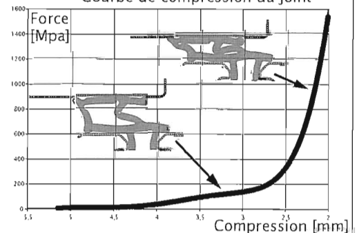
Courbe de compression du joint
