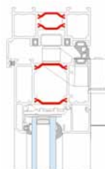
VERT. DOORSNEDE - COUPE VERTICALE
