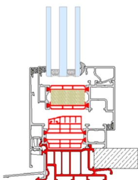
Basis profiel verdoken ontwatering Profil d'appui isolante drainage invisible
