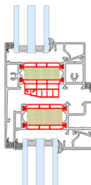
T-profiel bovenlicht Traverse imposte
